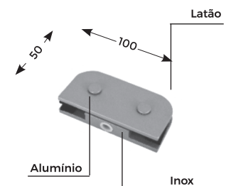
DOBRADIÇA PARA BASCULANTE 50x100
