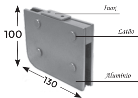
MAX DOBRADIÇA PIVOTANTE SUPERIOR COM PIVOT 1009 (AÇO INOX)
