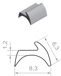
GUARNIÇÃO CUNHA PARA VIDRO
