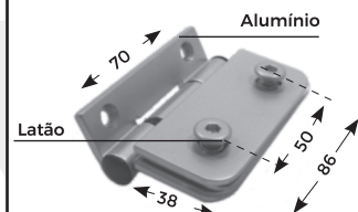
DOBRADIÇA PARA MAXIM-AR V/A (50mm ENTRE FUROS)
