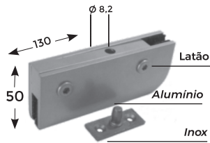
DOBRADIÇA PIVOTANTE SUPERIOR COM PIVOT 1009 (AÇO INOX)
