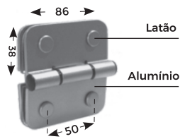
DOBRADIÇA PARA MAXIM-AR V/V (50mm ENTRE FUROS)
