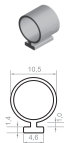
GUARNIÇÃO DO BATENTE
