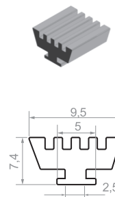
GUARNIÇÃO DA COLUNA E POLICARBONATO
