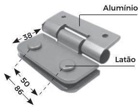
DOBRADIÇA (NÃO AUTOMÁTICA) PARA BOX
