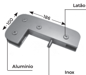
FACÃO SIMPLES COM PINO (AÇO INOX) PARA BANDEIRA E FIXO
