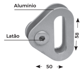
MINI PUXADOR DUPLO PARA TRANPASSE EM PORTAS E JANELA COM 1 FURO
