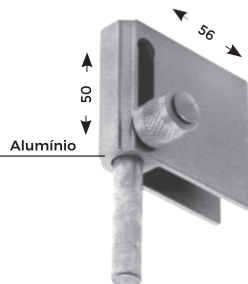
TRINCO DE PRESSÃO PARA JANELA DE CORRER FRONTAL
