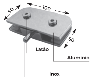
DOBRADIÇA COM PINO PARA BASCULANTE 50x100
