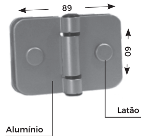
DOBRADIÇA DUPLA PARA JANELA
