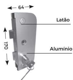
FECHADURA DE CENTRO COM 2 CILINDROS SEM MAÇANETA
