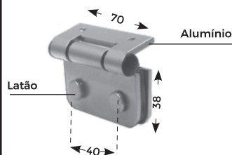
DOBRADIÇA PARA MAXIM-AR V/A (40mm ENTRE FUROS)
