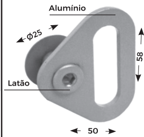
MINI PUXADOR PARA TRANPASSE EM PORTAS E JANELAS COM 1 FURO
