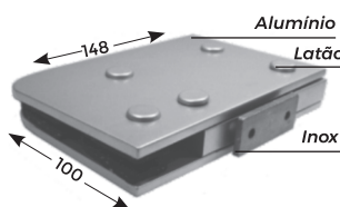
MAX DOBRADIÇA PIVOTANTE INFERIOR COM PIVOT 1014 (AÇO INOX)
