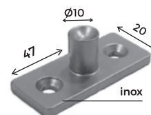
PIVOT INFERIOR 1014 (AÇO INOX)
