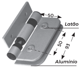
DOBRADIÇA AUTOMÁTICA PARA BOX
