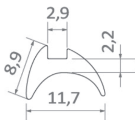
GUARNIÇÃO CUNHA PARA VIDRO
