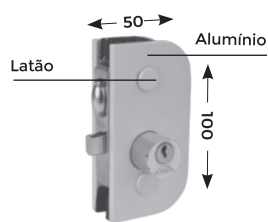
FECHADURA DE CENTRO COM ROLETE
