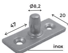
PIVOT SUPERIOR 1009 (AÇO INOX)
