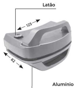
CONTRA FECHADURA PARA PORTA DE CORRER FURAÇÃO BLINDEX 1510BX
