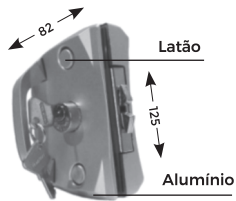
FECHADURA PARA PORTA DE CORRER FURAÇÃO BLINDEX 3530
