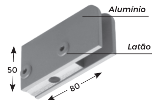
MINI DOBRADIÇA PIVOTANTE INFERIOR COM PIVOT 1014 (AÇO INOX)
