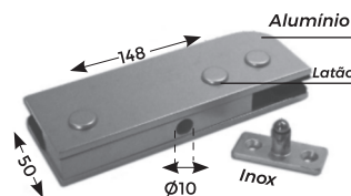
DOBRADIÇA PIVOTANTE INFERIOR COM PIVOT 1014 (AÇO INOX)
