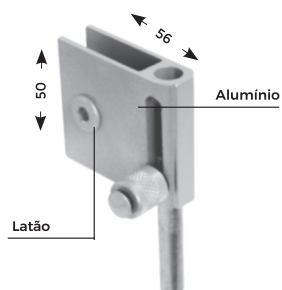
TRINCO PARA JANELA DE CORRER FRONTAL
