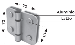
DOBRADIÇA PARA MAXIM-AR V/V (40mm ENTRE FUROS)
