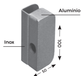
CONTRA FECHADURA DE PRESSÃO PARA 1520 P
